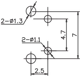
安装孔位图
